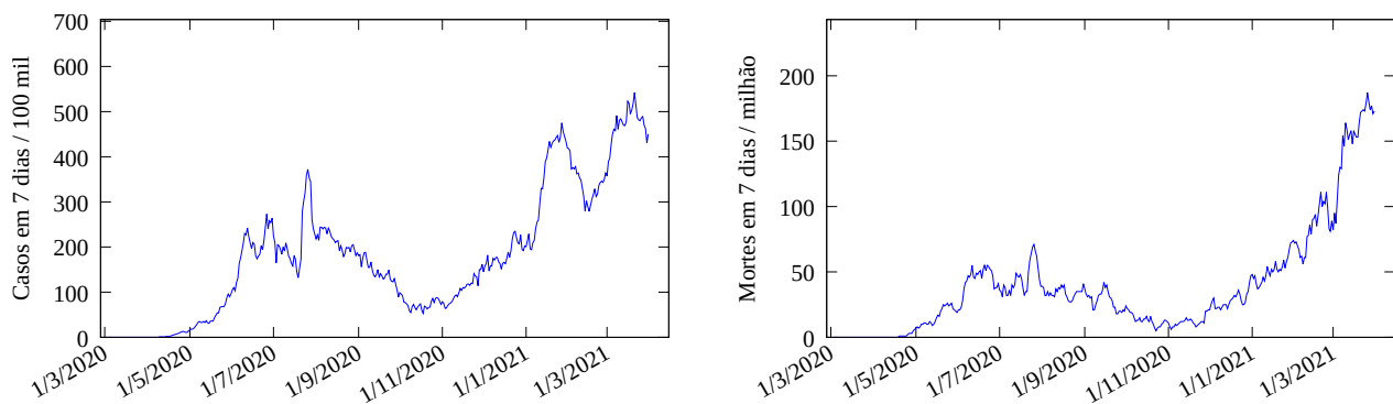
Figura 1: Esquerda: Casos novos de COVID-19 para cada 100 mil habitantes em Rondônia em função da data, com dados atualizados em 1/4/2021. Direita: Mortes para cada milhão de habitantes nos sete dias anteriores em Rondônia.
