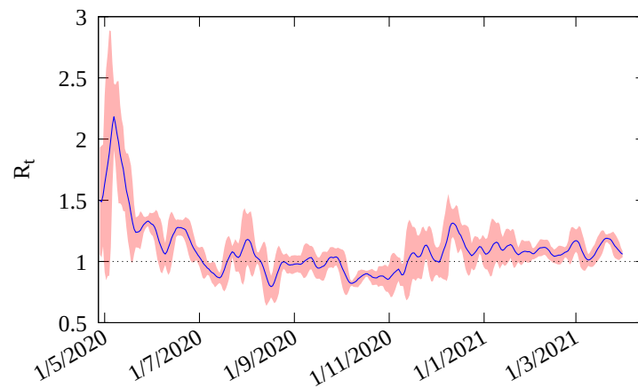
Figura 4: Número de reprodução básico R_t a partir do número de mortes em Rondônia , até a data de 1/4/2021 . O valor atual é de 1.06 .
