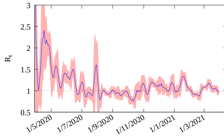
Figura 3: Número de reprodução básico R_t em Rondônia até a data de 1/4/2021 . O valor atual é de 0.95 .
