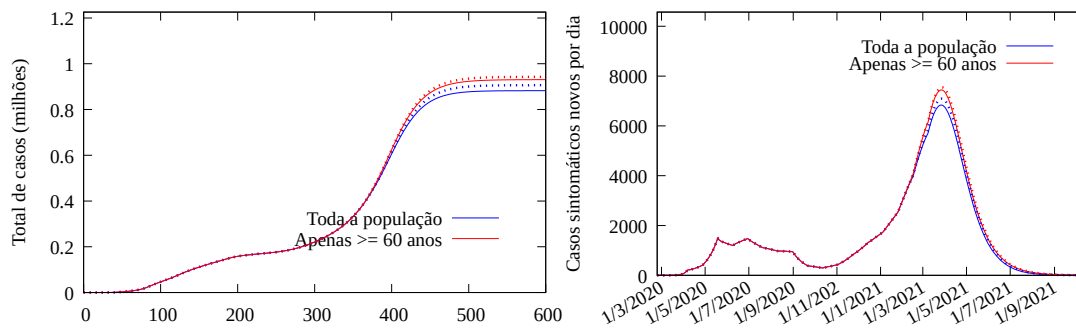
Figura 8: Esquerda: Modelo ajustado até o presente e prognósticos: estimativa do total real de casos sintomáticos em Rondônia . Direita: casos sintomáticos novos por dia.
