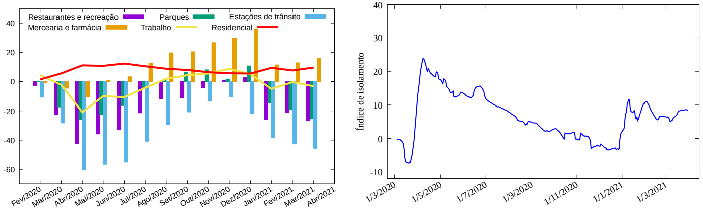
Figura 5: Esquerda: Variação percentual do tempo de permanência em cada categoria medida pela Google em Rondônia . Direita: Índice de isolamento (vide texto).
