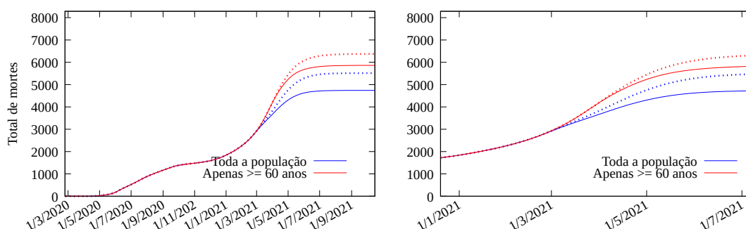
Figura 7: Modelo ajustado até o presente e prognósticos: total de mortes em Rondônia por COVID-19. O gráfico à direita é uma ampliação sobre o ano de 2021. A linha contínua em azul corresponde ao cenário em que toda a população é vacinada, começando pelos mais velhos (95% de eficácia linha contínua e 70% de eficácia linha pontilhada). A linha em vermelho corresponde ao cenário em que apenas pessoas com 60 anos ou mais de idade são vacinadas (95% de eficácia linha contínua e 70% de eficácia linha pontilhada).
