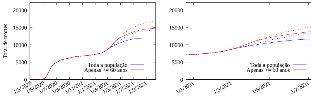
Figura 7: Modelo ajustado até o presente e prognósticos: total de mortes no Pará por COVID-19. O gráfico à direita é uma ampliação sobre o ano de 2021. A linha contínua em azul corresponde ao cenário em que toda a população é vacinada, começando pelos mais velhos (95% de eficácia linha contínua e 70% de eficácia linha pontilhada). A linha em vermelho corresponde ao cenário em que apenas pessoas com 60 anos ou mais de idade são vacinadas (95% de eficácia linha contínua e 70% de eficácia linha pontilhada).
