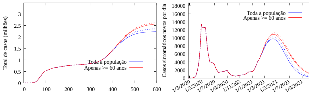
Figura 8: Esquerda: Modelo ajustado até o presente e prognósticos: estimativa do total real de casos sintomáticos no Pará. Direita: casos sintomáticos novos por dia.
