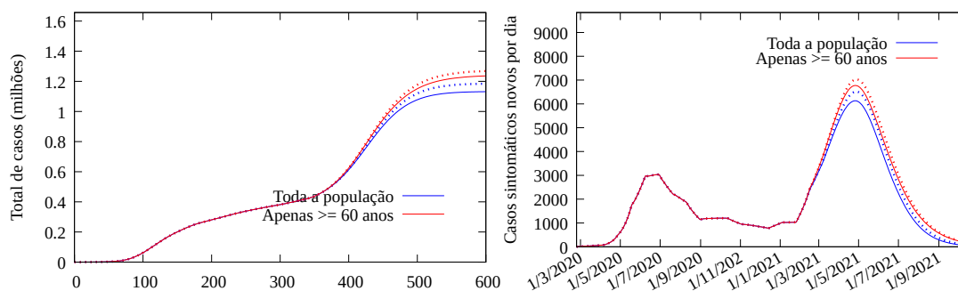
Figura 8: Esquerda: Modelo ajustado até o presente e prognósticos: estimativa do total real de casos sintomáticos no Piauí . Direita: casos sintomáticos novos por dia.
