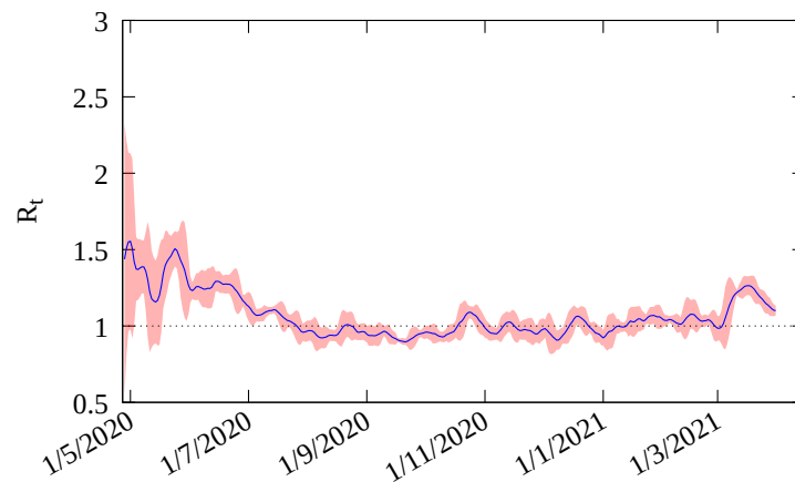
Figura 4: Número de reprodução básico R_t a partir do número de mortes no Piauí , até a data de 1/4/2021 . O valor atual é de 1.1 .
