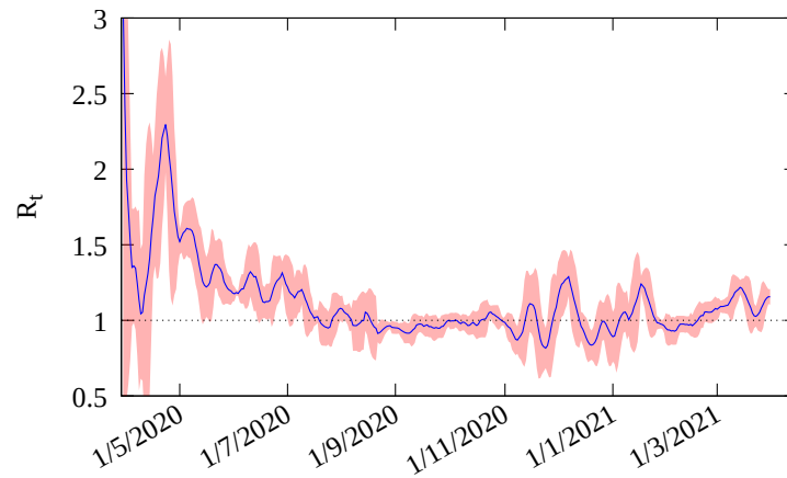
Figura 3: Número de reprodução básico R_t no Piauí até a data de 1/4/2021 . O valor atual é de 1.16
