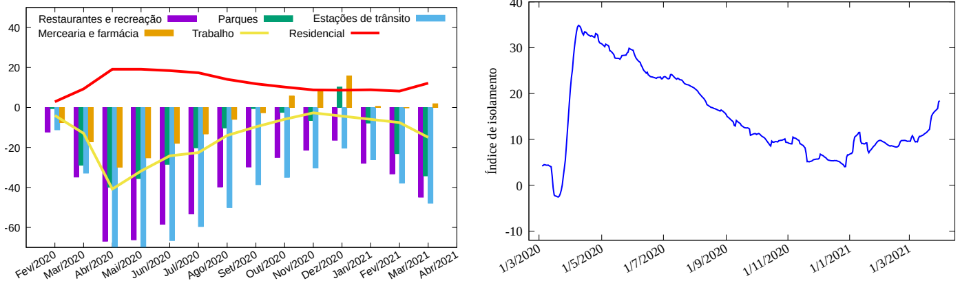
Figura 5: Esquerda: Variação percentual do tempo de permanência em cada categoria medida pela Google no Piauí . Direita: Índice de isolamento (vide texto).
