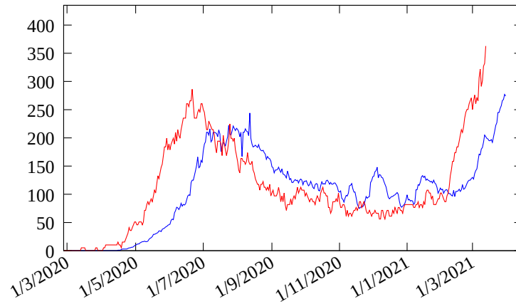
Figura 2: Série de casos por 100 mil habitantes e de mortes por milhão reescalada (ver texto).
