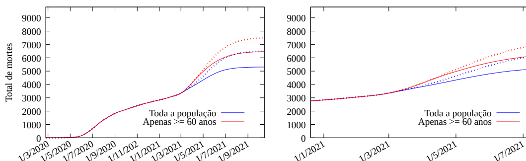
Figura 7: Modelo ajustado até o presente e prognósticos: total de mortes no Piauí por COVID-19. O gráfico à direita é uma ampliação sobre o ano de 2021. A linha contínua em azul corresponde ao cenário em que toda a população é vacinada, começando pelos mais velhos (95% de eficácia linha contínua e 70% de eficácia linha pontilhada). A linha em vermelho corresponde ao cenário em que apenas pessoas com 60 anos ou mais de idade são vacinadas (95% de eficácia linha contínua e 70% de eficácia linha pontilhada).
