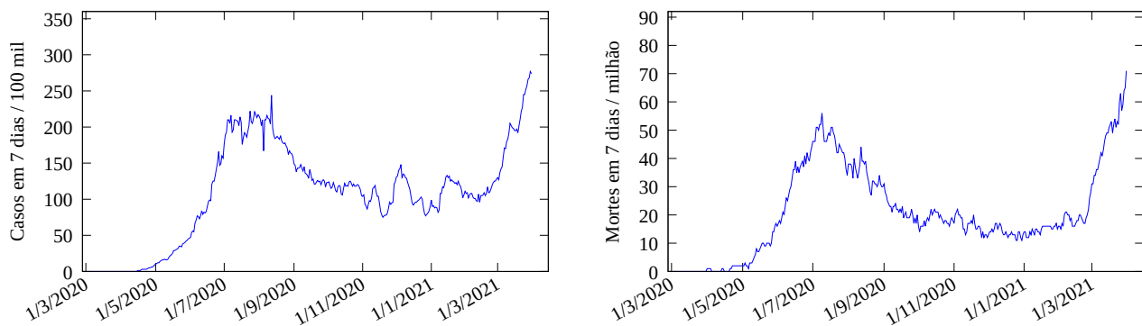
Figura 1: Esquerda: Casos novos de COVID-19 para cada 100 mil habitantes no Piauí em função da data, com dados atualizados em 1/4/2021. Direita: Mortes para cada milhão de habitantes nos sete dias anteriores no Piauí.
