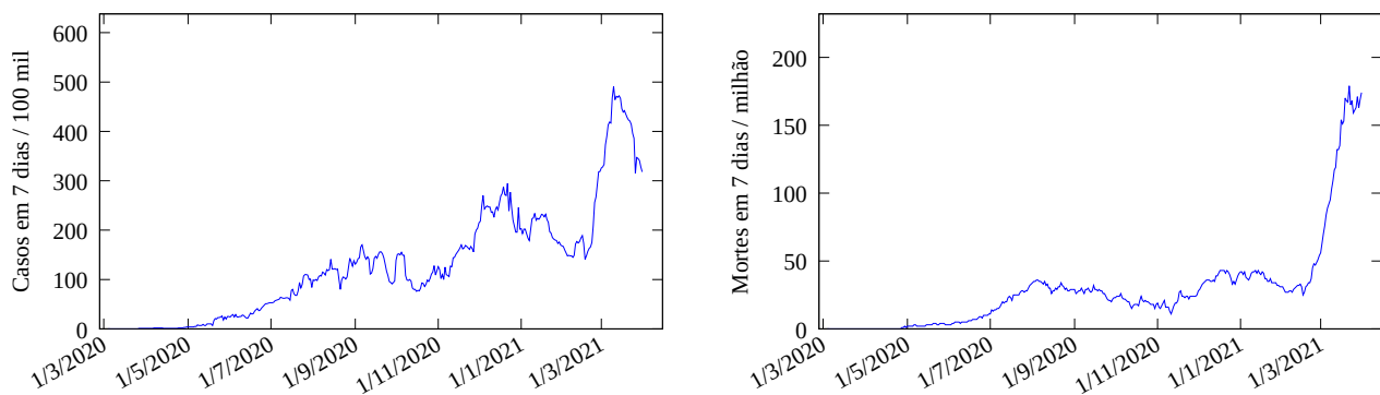
Figura 1: Esquerda: Casos novos de COVID-19 para cada 100 mil habitantes no Rio Grande do Sul em função da data, com dados atualizados em 1/4/2021. Direita: Mortes para cada milhão de habitantes nos sete dias anteriores no Rio Grande do Sul.
