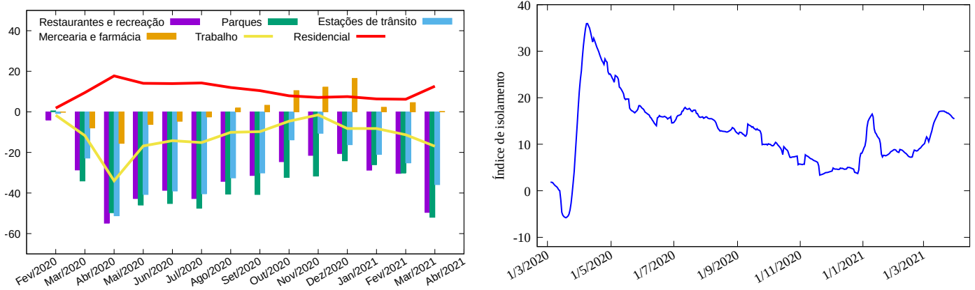
Figura 5: Esquerda: Variação percentual do tempo de permanência em cada categoria medida pela Google no Rio Grande do Sul. Direita: Índice de isolamento (vide texto).
