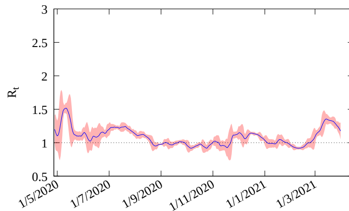
Figura 4: Número de reprodução básico R_t a partir do número de mortes no Rio Grande do Sul , até a data de 1/4/2021 . O valor atual é de 1.18 .
