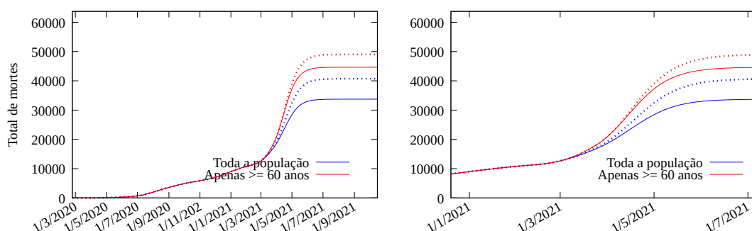
Figura 7: Modelo ajustado até o presente e prognósticos: total de mortes no Rio Grande do Sul por COVID-19. O gráfico à direita é uma ampliação sobre o ano de 2021. A linha contínua em azul corresponde ao cenário em que toda a população é vacinada, começando pelos mais velhos (95% de eficácia linha contínua e 70% de eficácia linha pontilhada). A linha em vermelho corresponde ao cenário em que apenas pessoas com 60 anos ou mais de idade são vacinadas (95% de eficácia linha contínua e 70% de eficácia linha pontilhada).
