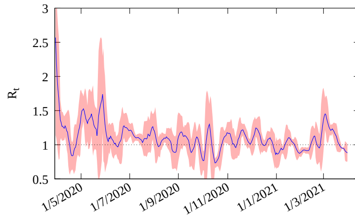
Figura 3: Número de reprodução básico R_t no Rio Grande do Sul até a data de 1/4/2021 . O valor atual é de 0.88 .
