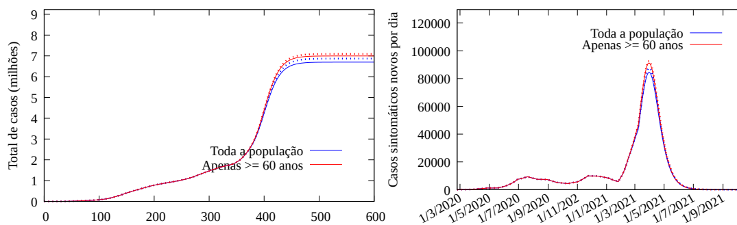
Figura 8: Esquerda: Modelo ajustado até o presente e prognósticos: estimativa do total real de casos sintomáticos no Rio Grande do Sul . Direita: casos sintomáticos novos por dia.
