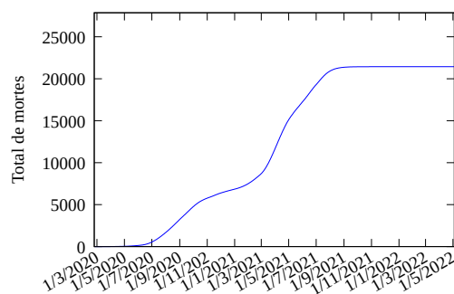
Figura 7: Modelo ajustado até o presente e prognóstico para o total de mortes em Goiás por COVID-19.
