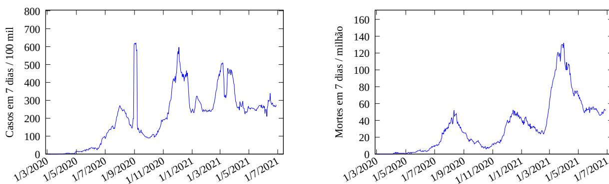
Figura 1: Esquerda: Casos novos de COVID-19 para cada 100 mil habitantes em Santa Catarina em função da data, com dados atualizados em 28/06/2021. Direita: Mortes para cada milhão de habitantes nos sete dias anteriores em Santa Catarina.
