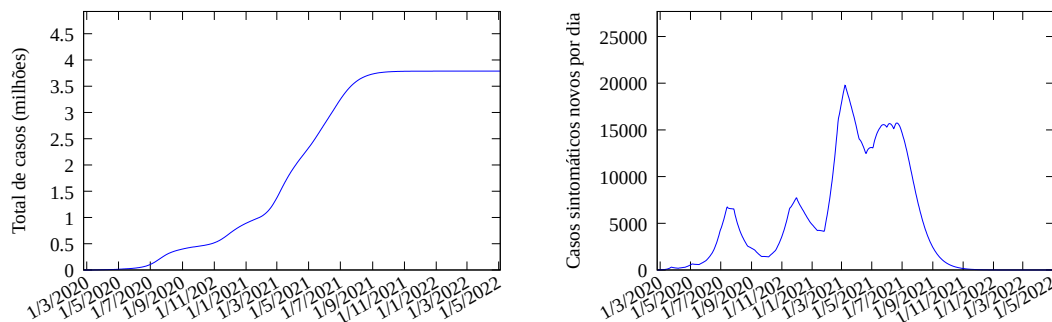
Figura 8: Esquerda: Modelo ajustado até o presente e prognósticos com a estimativa do total real de casos sintomáticos em Santa Catarina. Direita: casos sintomáticos novos por dia.
