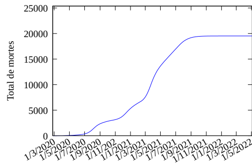
Figura 7: Modelo ajustado até o presente e prognóstico para o total de mortes em Santa Catarina por COVID-19.
