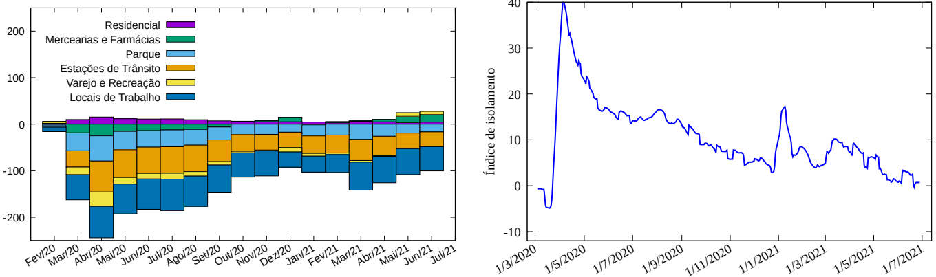
Figura 3: Esquerda: Variação percentual do tempo de permanência em cada categoria medida pela Google em Santa Catarina. Direita: Índice de isolamento (vide texto).
