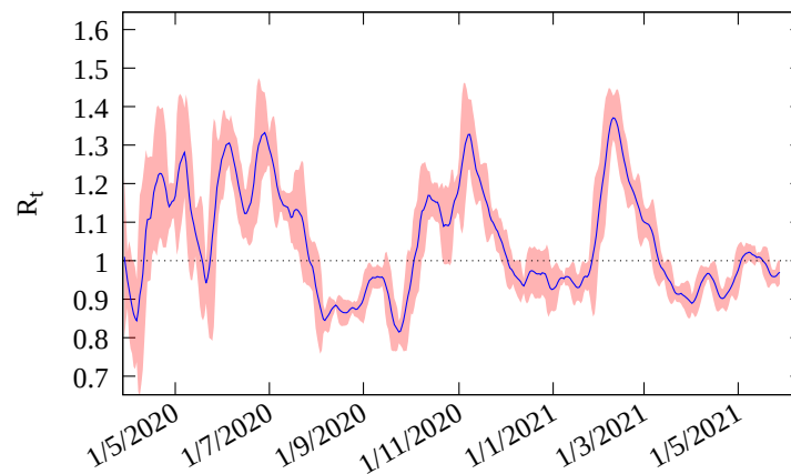
Figura 2: Número de reprodução básico R_t a partir do número total de mortes em Santa Catarina, até a data de 28/06/2021. O valor atual é de 0.97.
