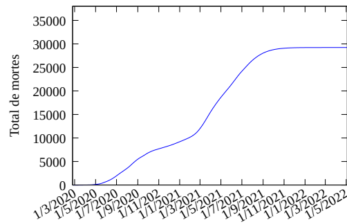
Figura 7: Modelo ajustado até o presente e prognóstico para o total de mortes na Bahia por COVID-19.
