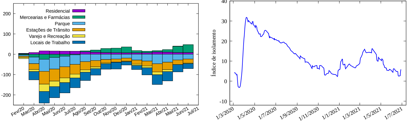
Figura 3: Esquerda: Variação percentual do tempo de permanência em cada categoria medida pela Google na Bahia . Direita: Índice de isolamento (vide texto).
