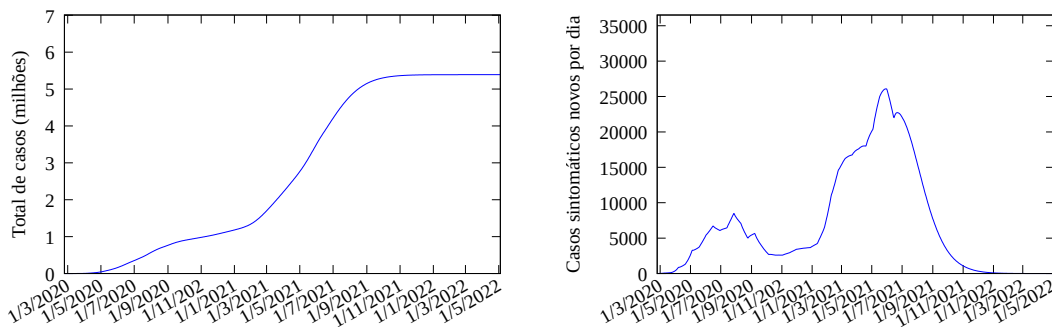
Figura 8: Esquerda: Modelo ajustado até o presente e prognósticos com a estimativa do total real de casos sintomáticos na Bahia. Direita: casos sintomáticos novos por dia.
