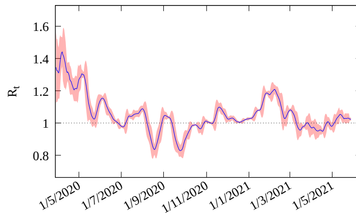
Figura 2: Número de reprodução básico R_t a partir do número total de mortes na Bahia , até a data de 28/06/2021 . O valor atual é de 1.02 .
