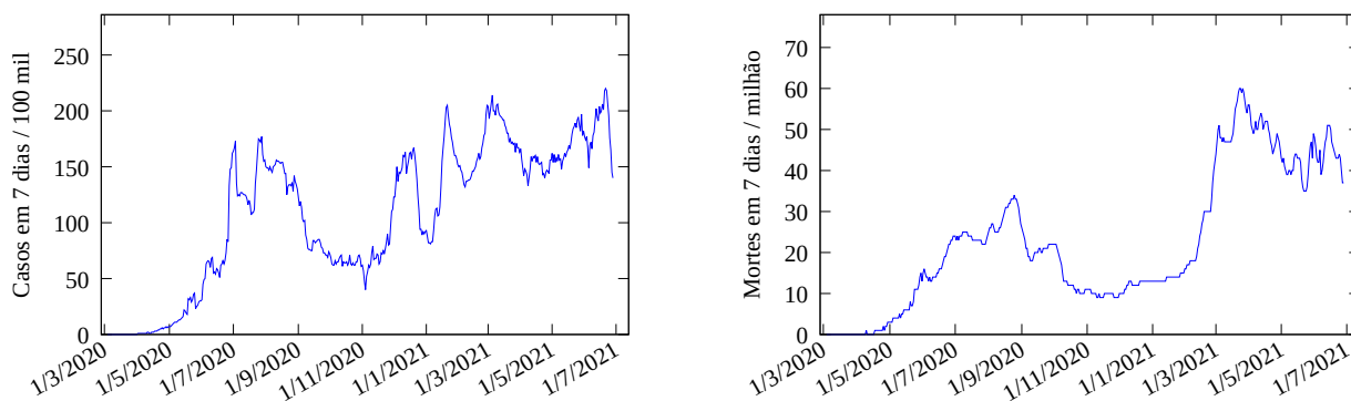
Figura 1: Esquerda: Casos novos de COVID-19 para cada 100 mil habitantes na Bahia em função da data, com dados atualizados em 28/06/2021. Direita: Mortes para cada milhão de habitantes nos sete dias anteriores na Bahia.
