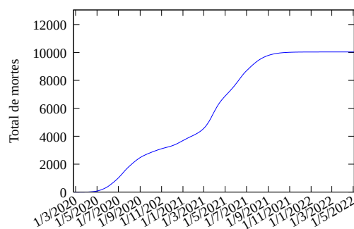
Figura 7: Modelo ajustado até o presente e prognóstico para o total de mortes na Paraíba por COVID-19.
