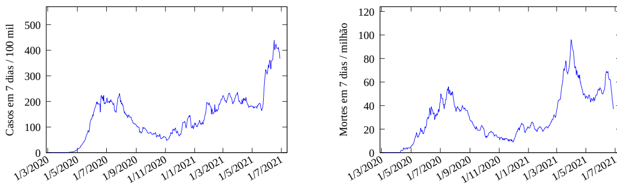
Figura 1: Esquerda: Casos novos de COVID-19 para cada 100 mil habitantes na Paraíba em função da data, com dados atualizados em 28/06/2021. Direita: Mortes para cada milhão de habitantes nos sete dias anteriores na Paraíba.
