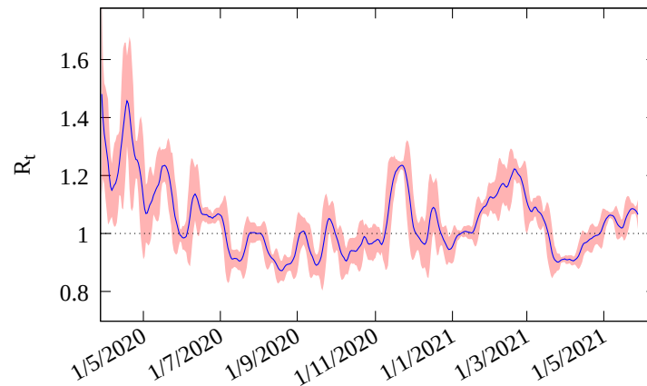
Figura 2: Número de reprodução básico R_t a partir do número total de mortes na Paraíba, até a data de 28/06/2021. O valor atual é de 1.07.
