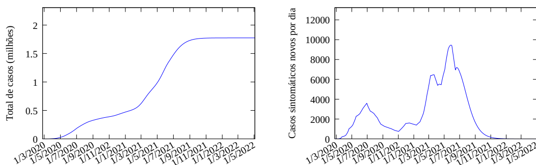
Figura 8: Esquerda: Modelo ajustado até o presente e prognósticos com a estimativa do total real de casos sintomáticos na Paraíba. Direita: casos sintomáticos novos por dia.
