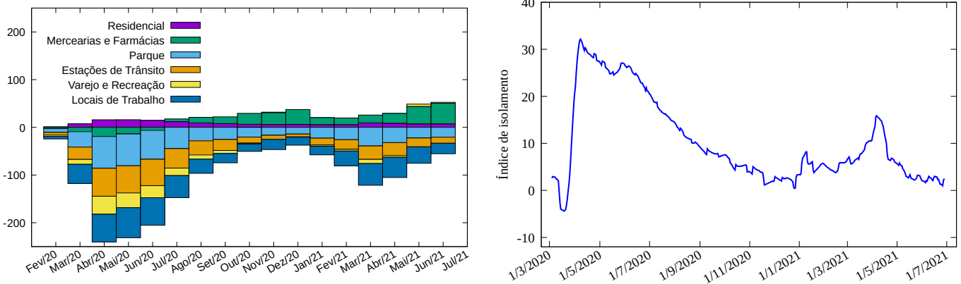
Figura 3: Esquerda: Variação percentual do tempo de permanência em cada categoria medida pela Google na Paraíba. Direita: Índice de isolamento (vide texto).
