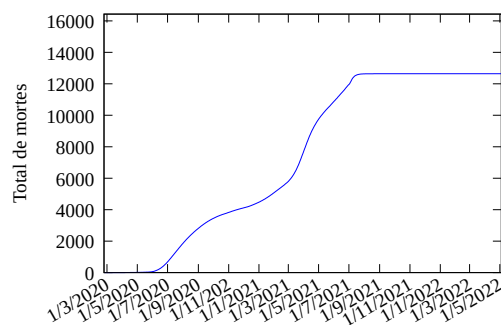
Figura 7: Modelo ajustado até o presente e prognóstico para o total de mortes no Mato Grosso por COVID-19.
