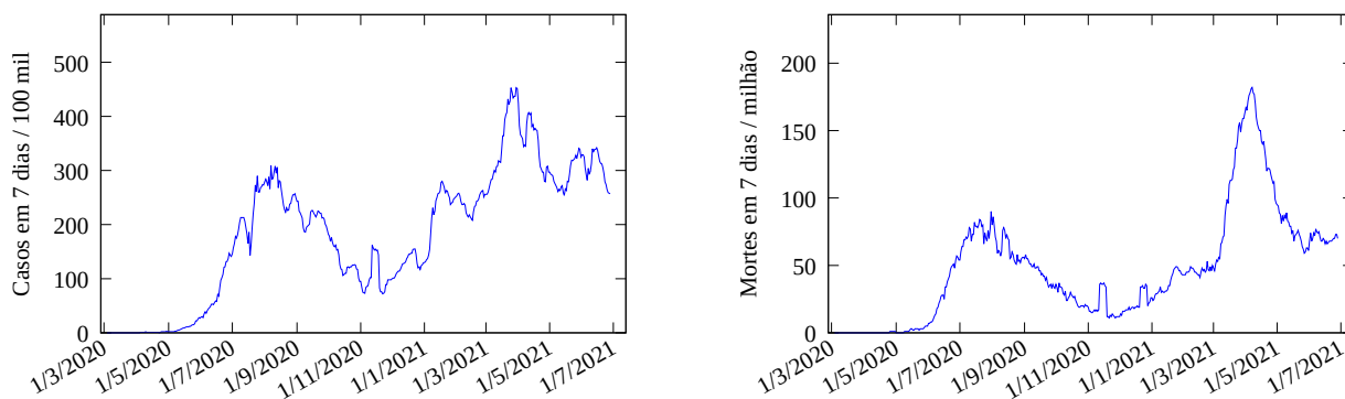
Figura 1: Esquerda: Casos novos de COVID-19 para cada 100 mil habitantes no Mato Grosso em função da data, com dados atualizados em 28/06/2021. Direita: Mortes para cada milhão de habitantes nos sete dias anteriores no Mato Grosso.
