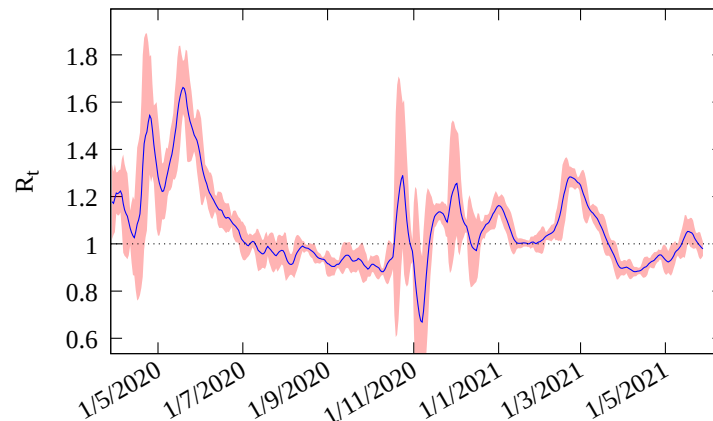
Figura 2: Número de reprodução básico R_t a partir do número total de mortes no Mato Grosso , até a data de 28/06/2021 . O valor atual é de 0.97 .
