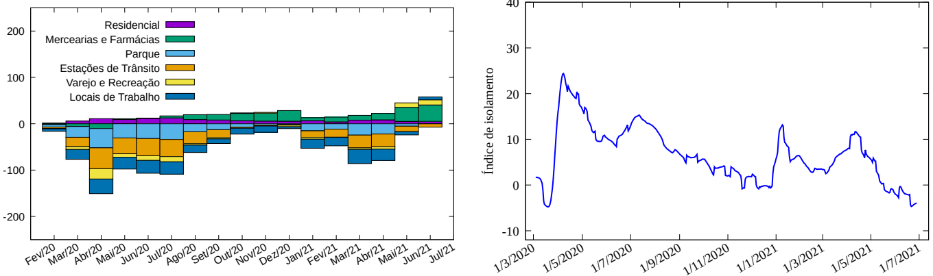
Figura 3: Esquerda: Variação percentual do tempo de permanência em cada categoria medida pela Google no Mato Grosso . Direita: Índice de isolamento (vide texto).
