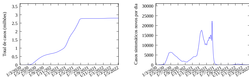
Figura 8: Esquerda: Modelo ajustado até o presente e prognósticos com a estimativa do total real de casos sintomáticos no Mato Grosso. Direita: casos sintomáticos novos por dia.
