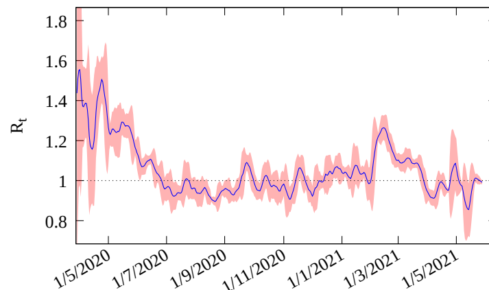
Figura 2: Número de reprodução básico R_t a partir do número total de mortes no Piauí , até a data de 28/06/2021 . O valor atual é de 0.99 .
