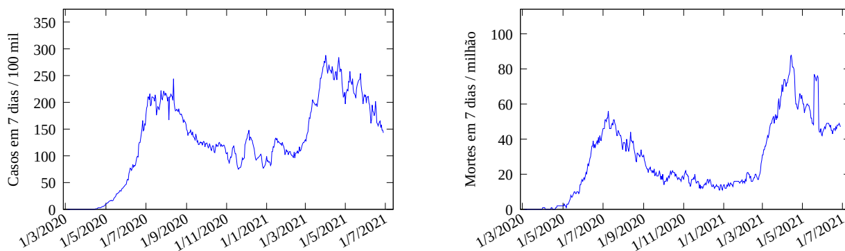
Figura 1: Esquerda: Casos novos de COVID-19 para cada 100 mil habitantes no Piauí em função da data, com dados atualizados em 28/06/2021. Direita: Mortes para cada milhão de habitantes nos sete dias anteriores no Piauí.
