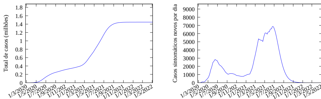
Figura 8: Esquerda: Modelo ajustado até o presente e prognósticos com a estimativa do total real de casos sintomáticos no Piauí. Direita: casos sintomáticos novos por dia.
