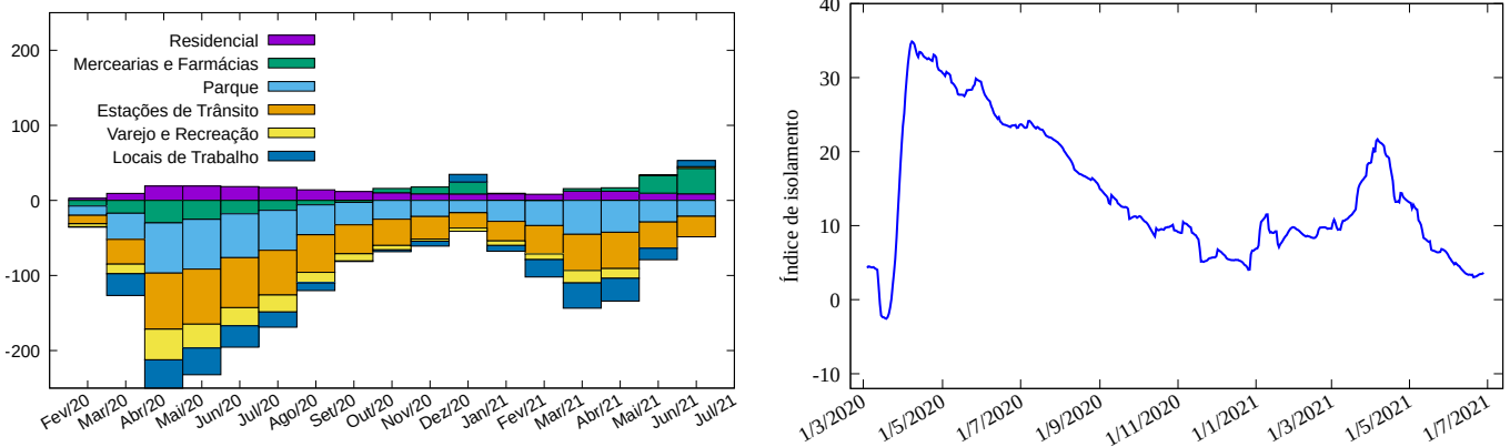
Figura 3: Esquerda: Variação percentual do tempo de permanência em cada categoria medida pela Google no Piauí. Direita: Índice de isolamento (vide texto).
