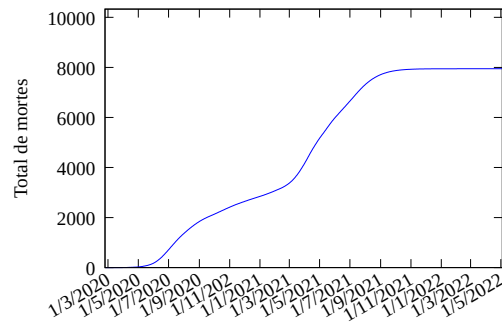
Figura 7: Modelo ajustado até o presente e prognóstico para o total de mortes no Piauí por COVID-19.
