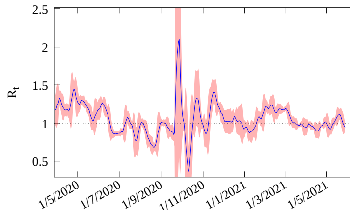
Figura 2: Número de reprodução básico R_t a partir do número total de mortes no Rio Grande do Norte, até a data de 28/06/2021. O valor atual é de 0.94.
