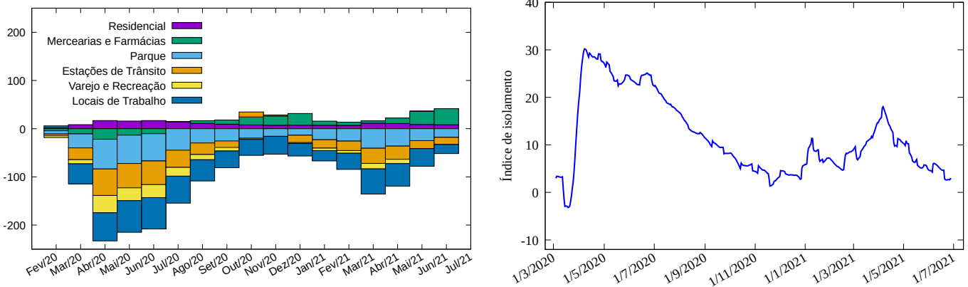
Figura 3: Esquerda: Variação percentual do tempo de permanência em cada categoria medida pela Google no Rio Grande do Norte . Direita: Índice de isolamento (vide texto).
