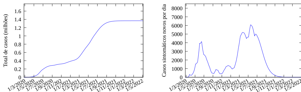
Figura 8: Esquerda: Modelo ajustado até o presente e prognósticos com a estimativa do total real de casos sintomáticos no Rio Grande do Norte. Direita: casos sintomáticos novos por dia.
