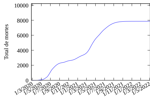
Figura 7: Modelo ajustado até o presente e prognóstico para o total de mortes no Rio Grande do Norte por COVID-19.
