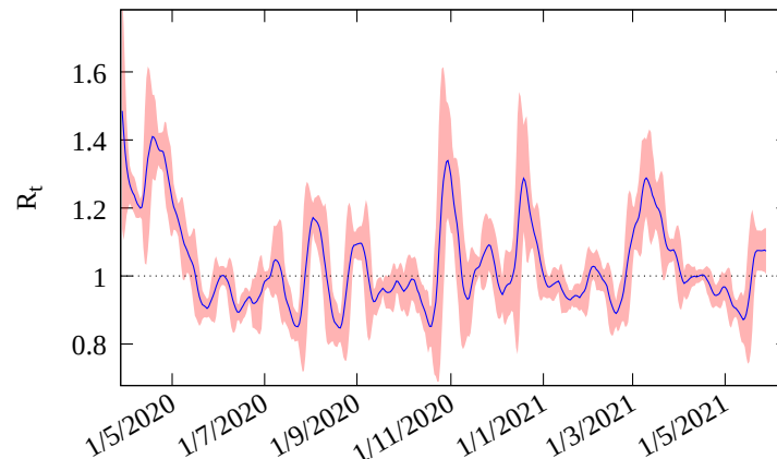
Figura 2: Número de reprodução básico R_t a partir do número total de mortes no Rio de Janeiro , até a data de 28/06/2021 . O valor atual é de 1.07 .
