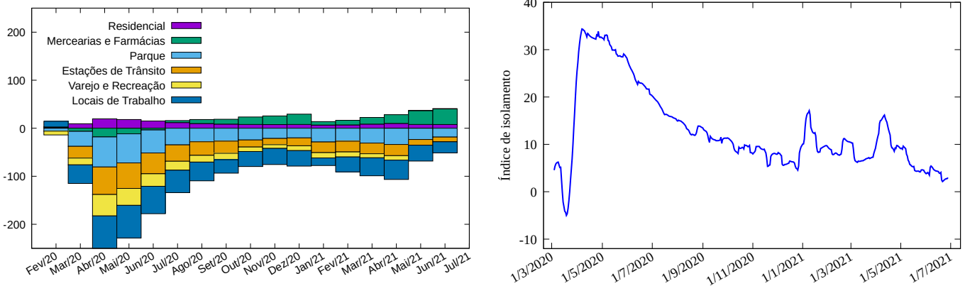
Figura 3: Esquerda: Variação percentual do tempo de permanência em cada categoria medida pela Google no Rio de Janeiro. Direita: Índice de isolamento (vide texto).
