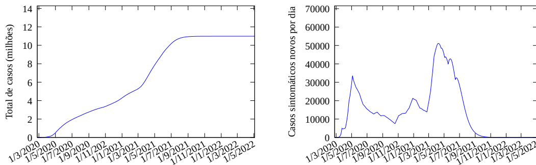
Figura 8: Esquerda: Modelo ajustado até o presente e prognósticos com a estimativa do total real de casos sintomáticos no Rio de Janeiro. Direita: casos sintomáticos novos por dia.
