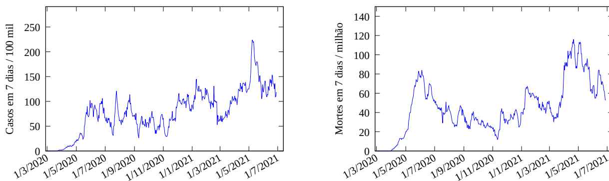
Figura 1: Esquerda: Casos novos de COVID-19 para cada 100 mil habitantes no Rio de Janeiro em função da data, com dados atualizados em 28/06/2021. Direita: Mortes para cada milhão de habitantes nos sete dias anteriores no Rio de Janeiro.
