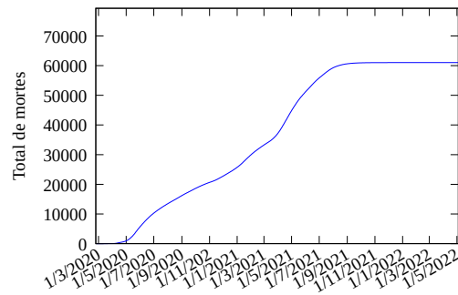
Figura 7: Modelo ajustado até o presente e prognóstico para o total de mortes no Rio de Janeiro por COVID-19.
